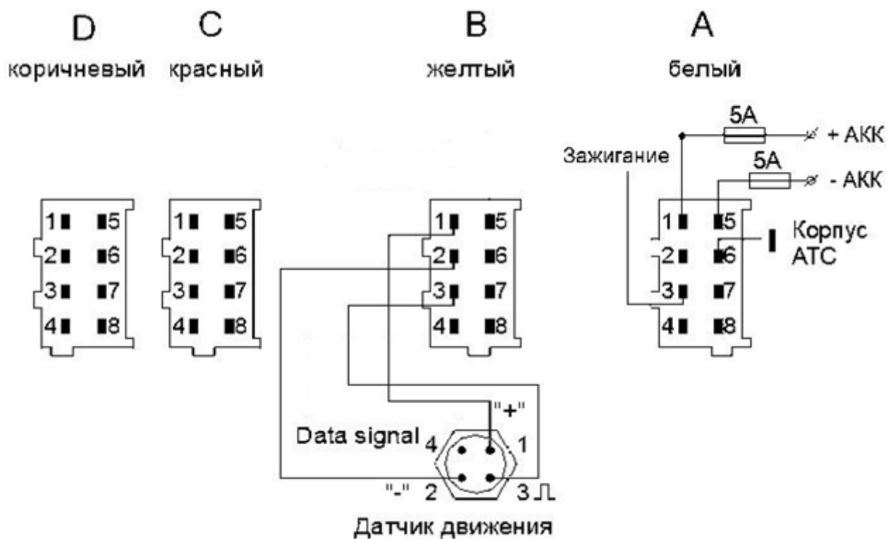
Рисунок 4. Схема подключения тахографа на ТС для перевозки опасных грузов
