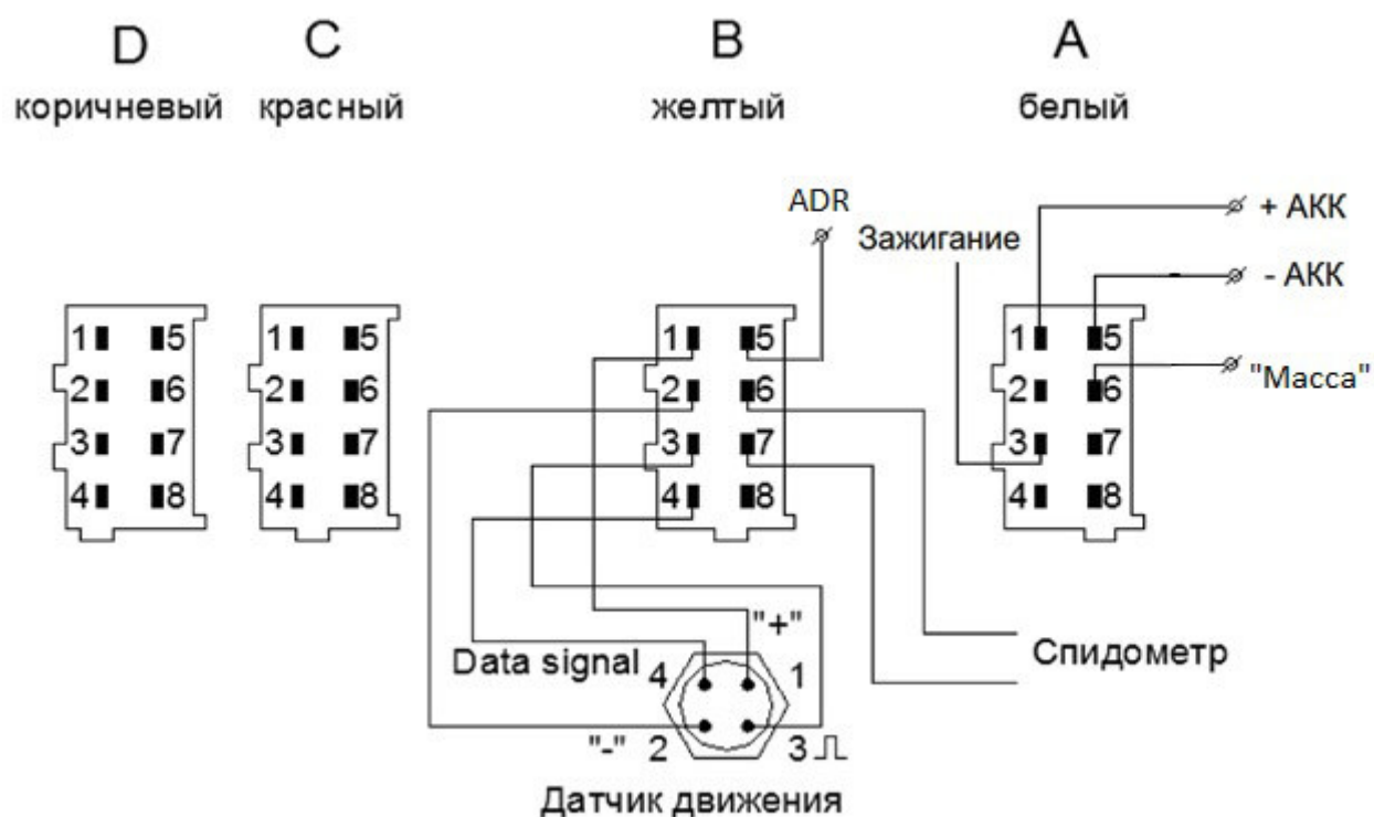
Рисунок 1. Схема подключения тахографа при использовании аналогового спидометра
