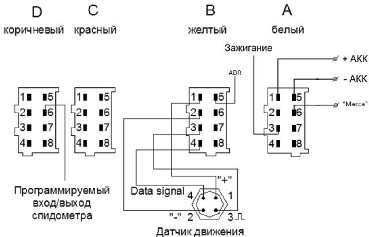
Рисунок 3. Схема подключения тахографа при использовании спидометра с программируемым входом
