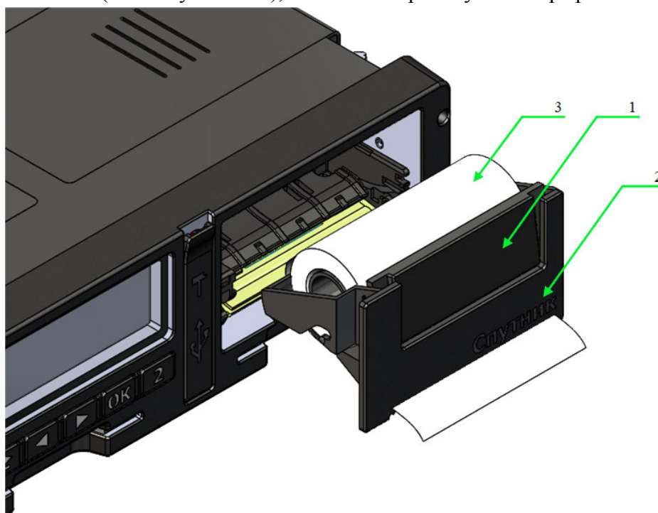
Рисунок 2.12 Замена бумаги в кассете термопринтера.
