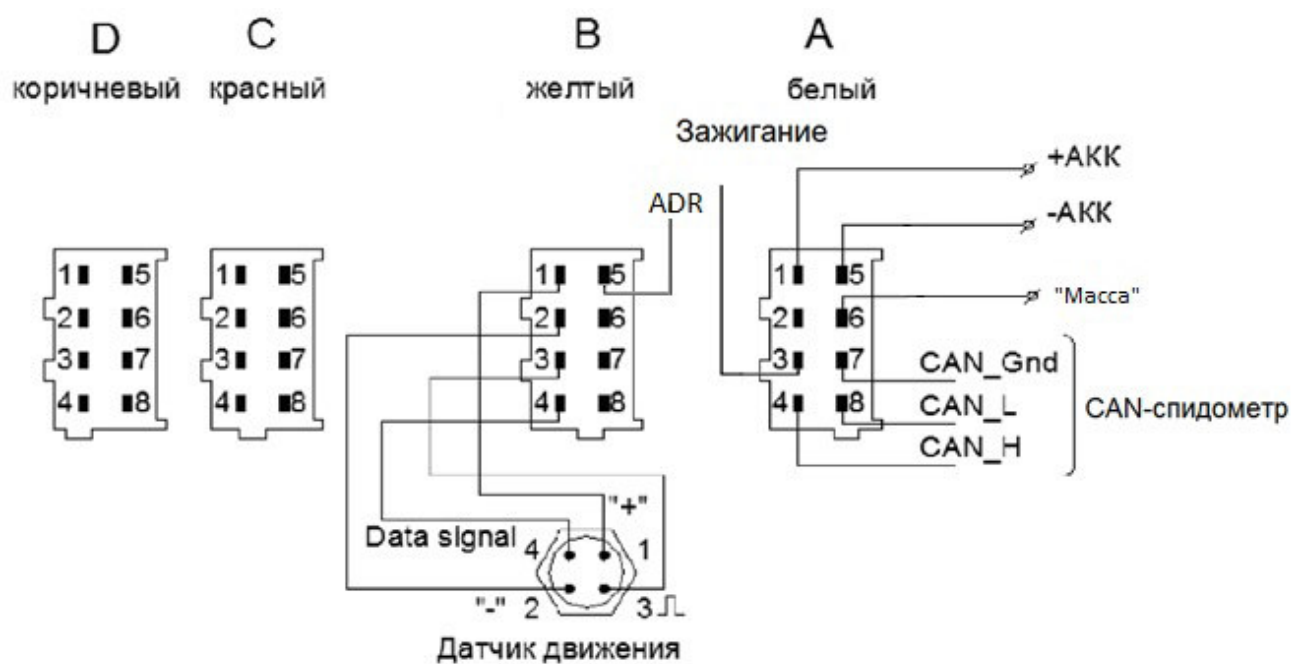
Рисунок 2. Схема подключения тахографа при использовании CAN-спидометра
